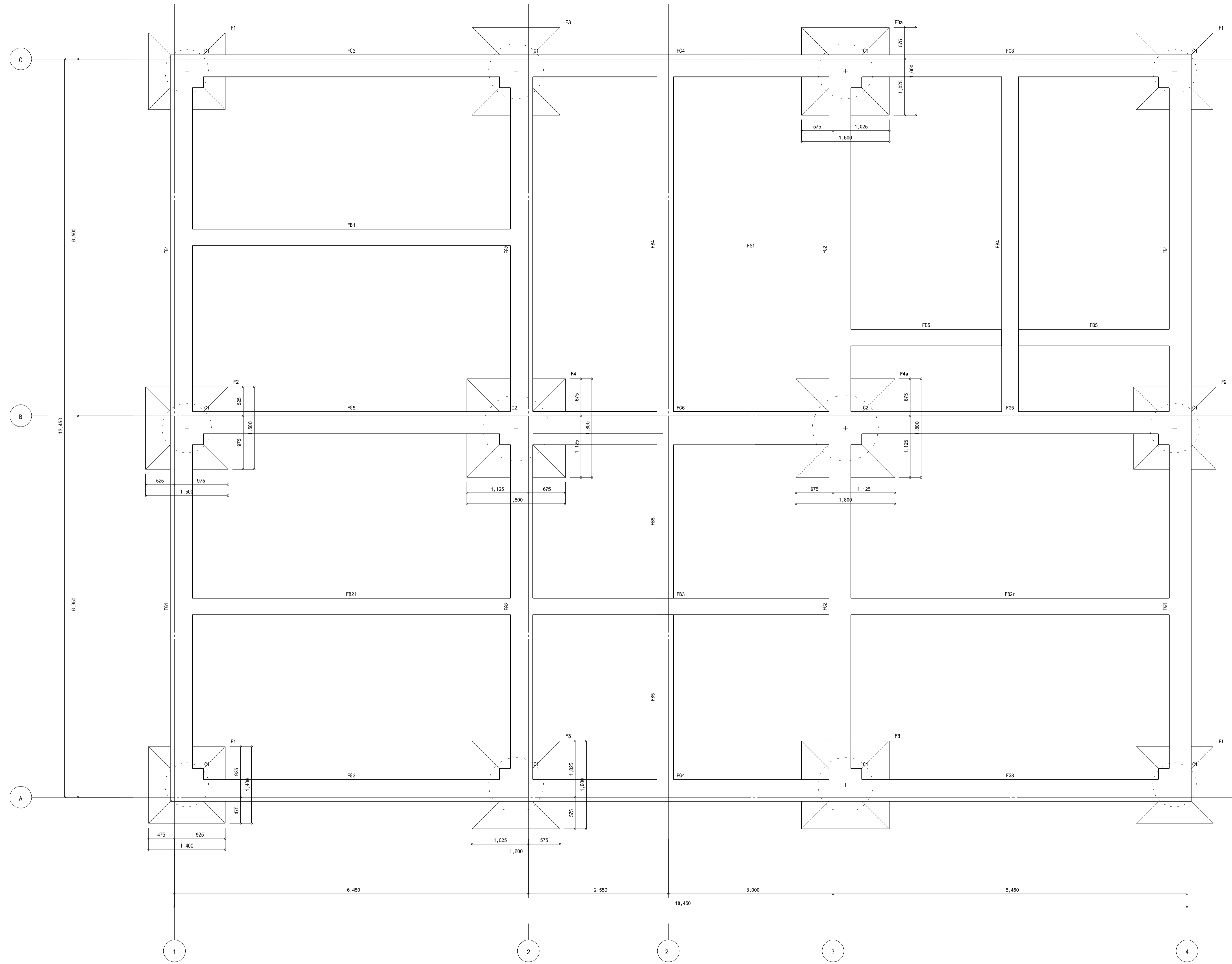
基礎伏図 1:40
