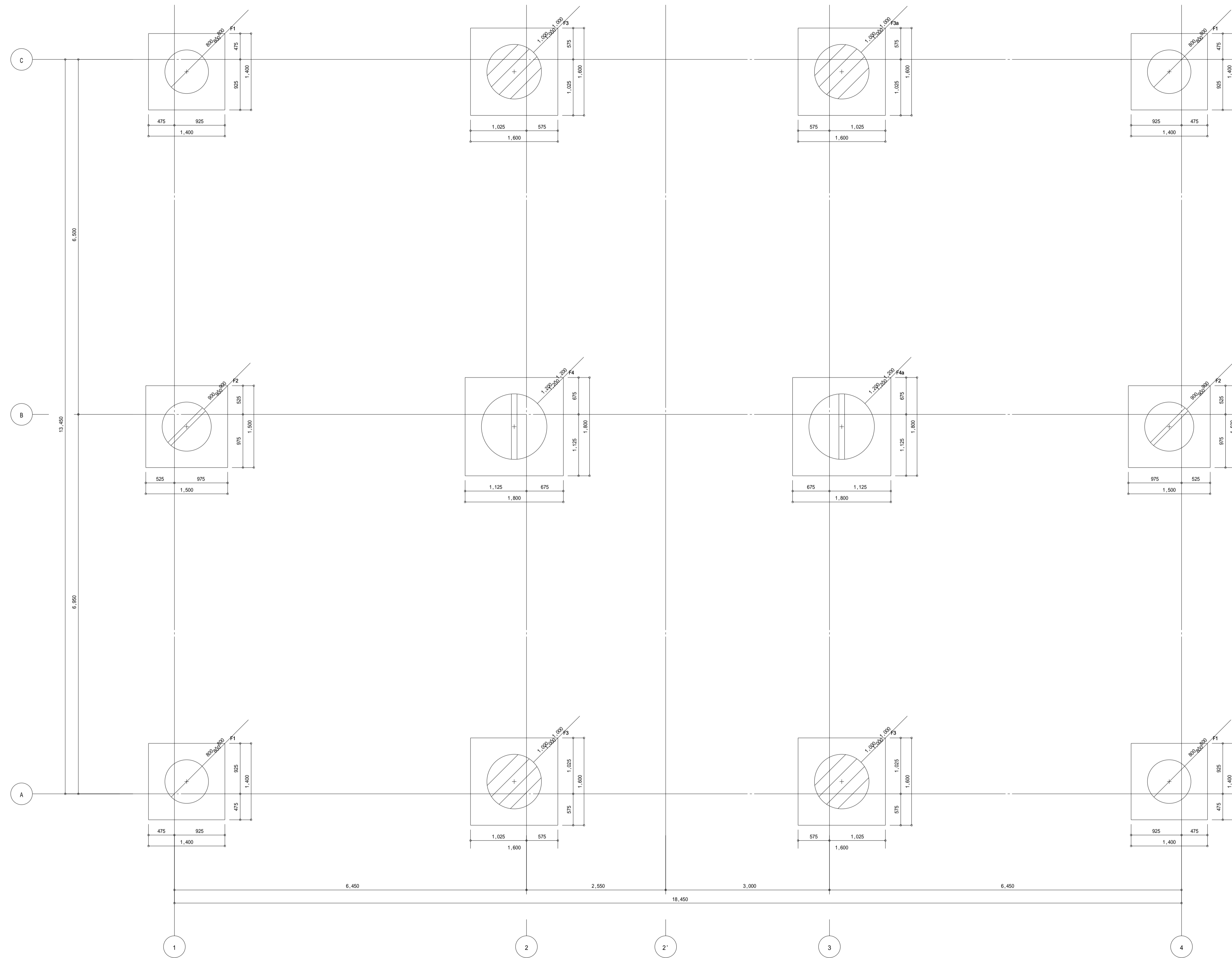
杭伏図 1:40
