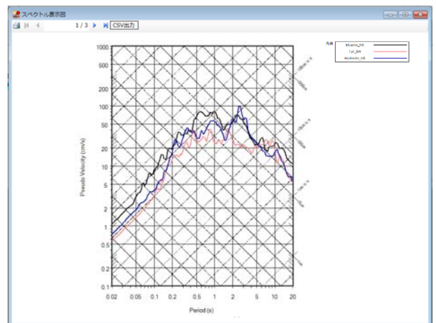
擬似速度応答スペクトル図
